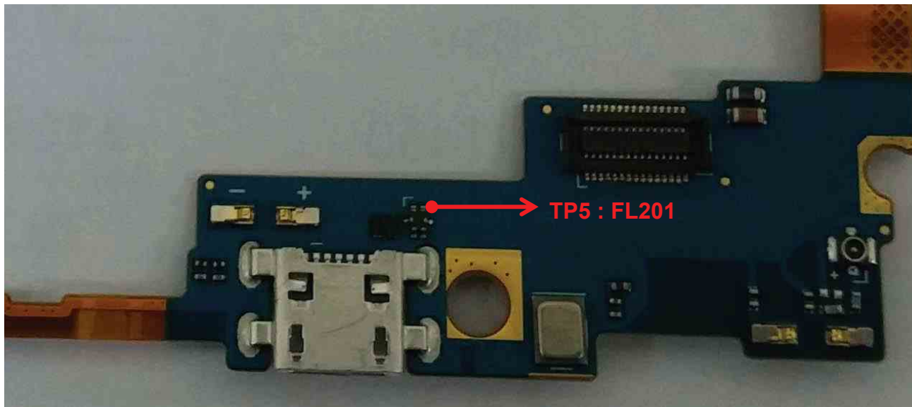
<Lower FPCB bot >
